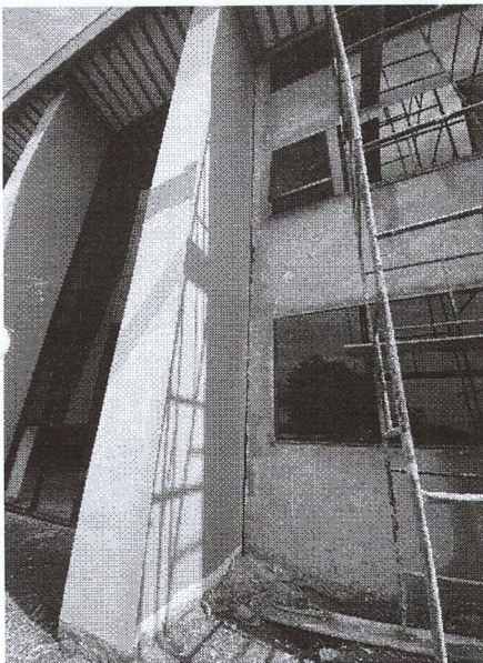
=> PELE DE VIDRO E TRATAMENTO DE JUNTA DE DILATAÇÃO NA FACHADA FRONTAL - COR CINZA
