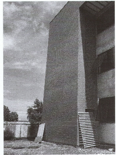
=> REVESTIMENTO EXTERNO COM LITOCERÂMICA - FACHADA FRONTAL ESQUERDA DETALHE
