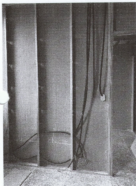
=> Térreo - Instalações Elétricas
