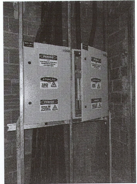
=> Quadro de distribuição e disjuntores - 1 Pavimento
